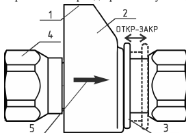
Рисунок 5. – Клапан КЗГЭМ-БМ.
