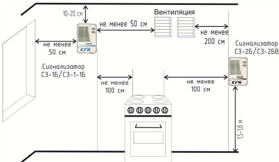
Рис.2 Схема размещение сигнализаторов загазованности СГК-СЗ.
