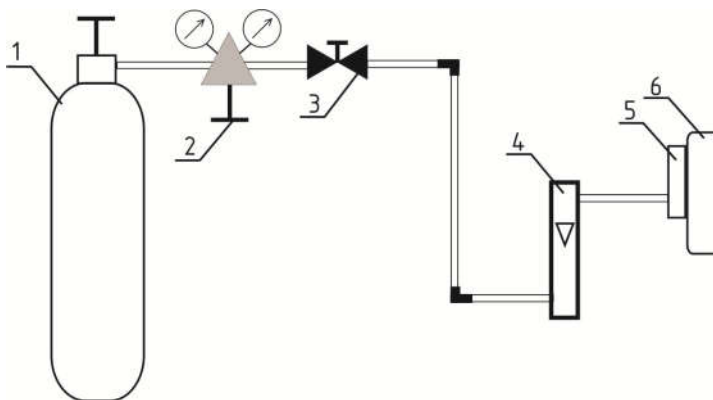
Рисунок Б.1 – Рекомендуемая схема подачи ГС на вход сигнализаторов загазованности бытовых СЗ-Б
