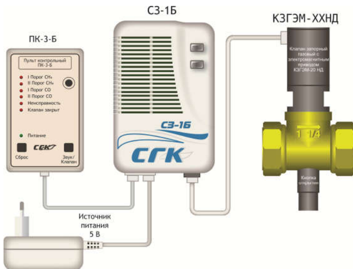
Рис.3. Сигнализаторы СЗ-Б с клапаном КЗГЭМ и пультом контрольным ПК-3-Б
