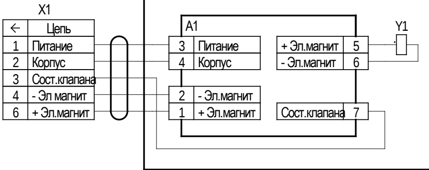
Рисунок Д.1 – Назначение контактов разъема у клапанов (СД) с разъемом РГ -17.
